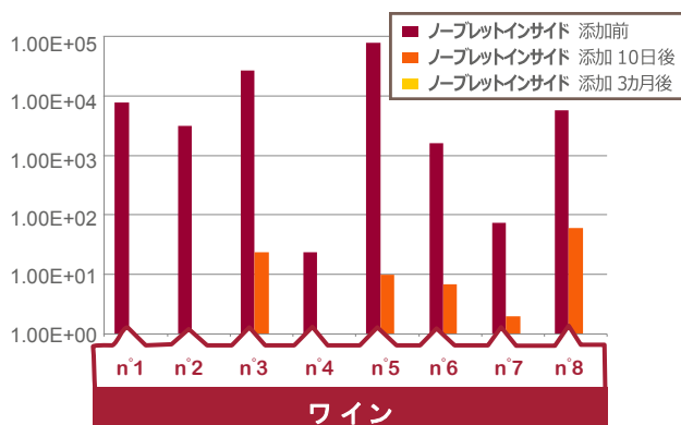
ブレタノマイセス菌数 (UFC/mL), RT-PCR
