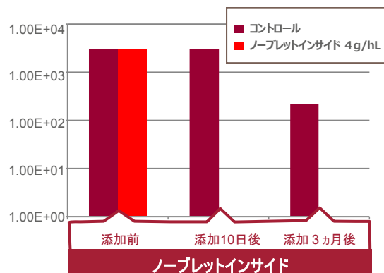
ブレタノマイセス菌数 (UFC/mL), RT-PCR
